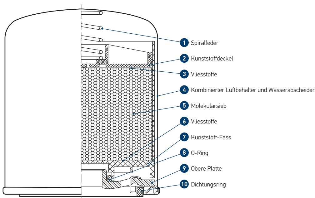
Produkt-Skizze
